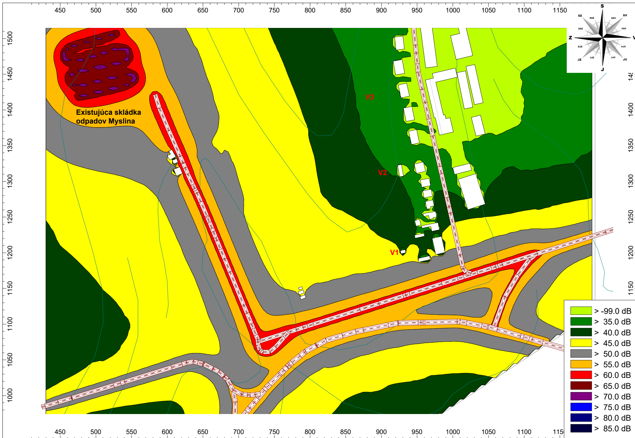
Príloha 2 - Matematický model (hluková mapa) záujmového územia "Skládka odpadov Myslina – Lúčky – CENTRUM MBÚ – Myslina" - súčasný stav - denný čas - výška izofón 3m nad povrchom terénu.
