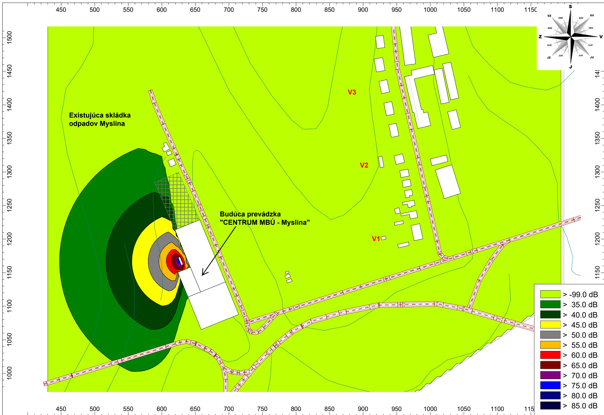
Príloha 4 - Matematický model (hluková mapa) záujmového územia "Skládka odpadov Myslina – Lúčky – CENTRUM MBÚ – Myslina" - predikcia - večerný čas - výška izofón 3m nad povrchom terénu.
