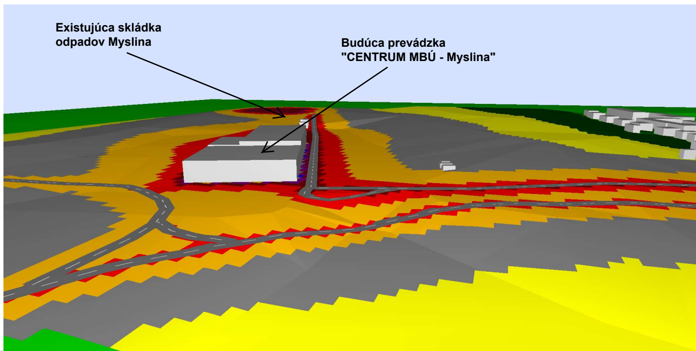
Príloha 1B - 3D pohľad matematického modelu (hlukovej mapy) záujmového územia "Skládka odpadov Myslina – Lúčky – CENTRUM MBÚ – Myslina" - denný čas - predikcia.
