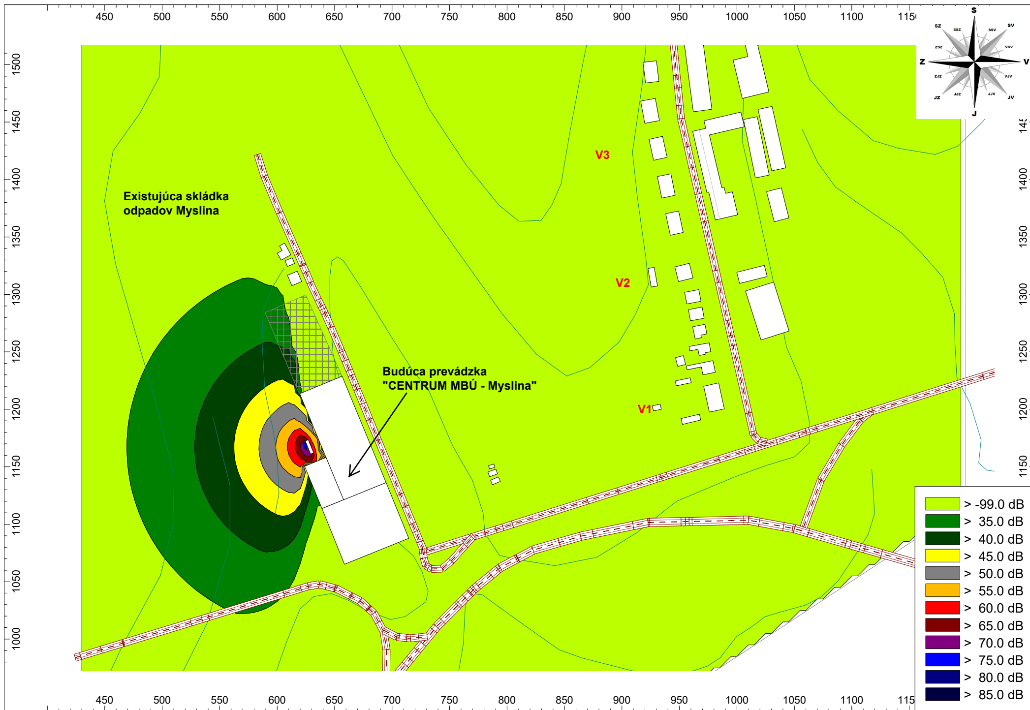
Príloha 5 - Matematický model (hluková mapa) záujmového územia "Skládka odpadov Myslina – Lúčky – CENTRUM MBÚ – Myslina" - predikcia - nočný čas - výška izofón 3m nad povrchom terénu.
