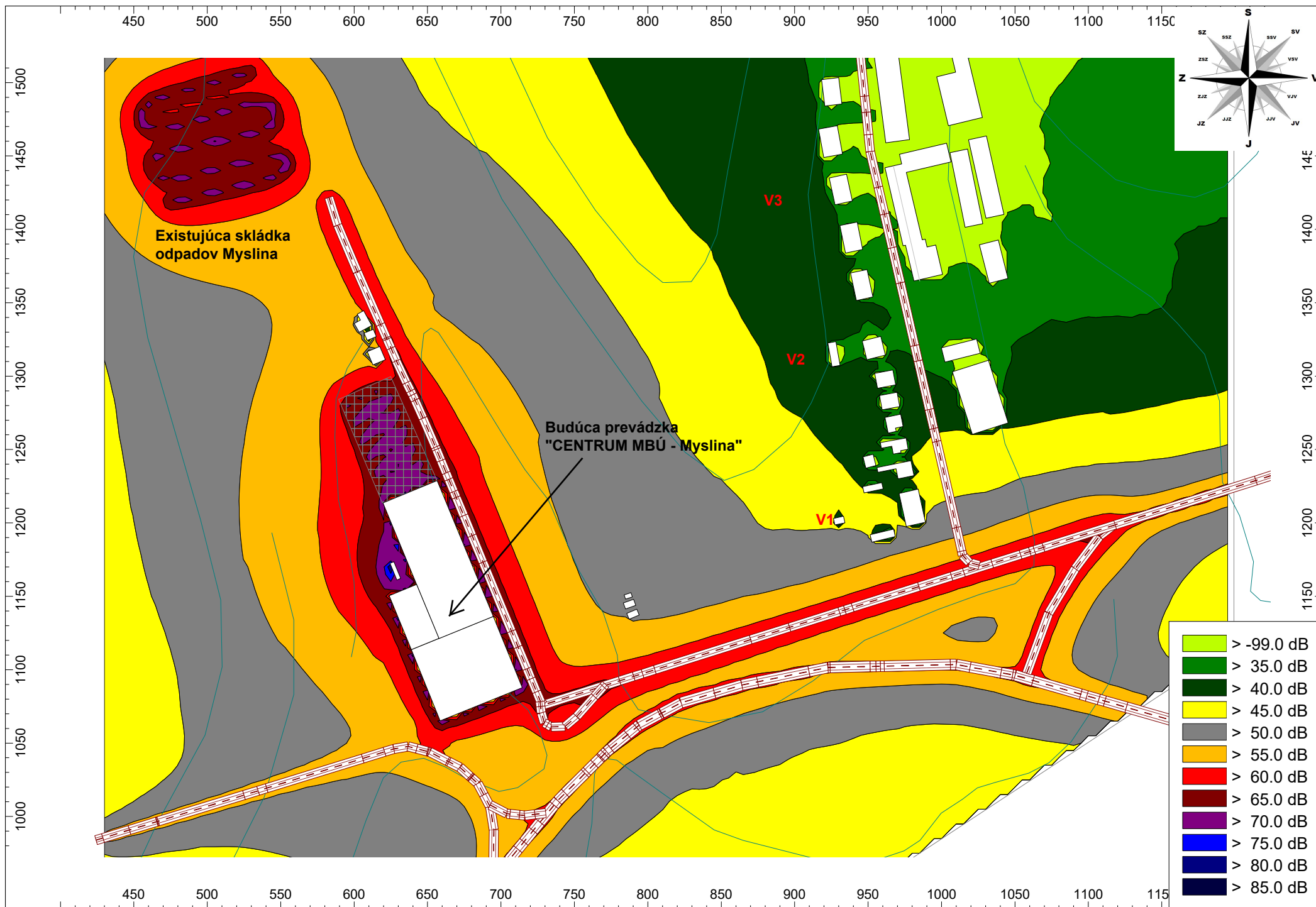
Príloha 3 - Matematický model (hluková mapa) záujmového územia "Skládka odpadov Myslina – Lúčky – CENTRUM MBÚ – Myslina" - predikcia - denný čas - výška izofón 3m nad povrchom terénu.
