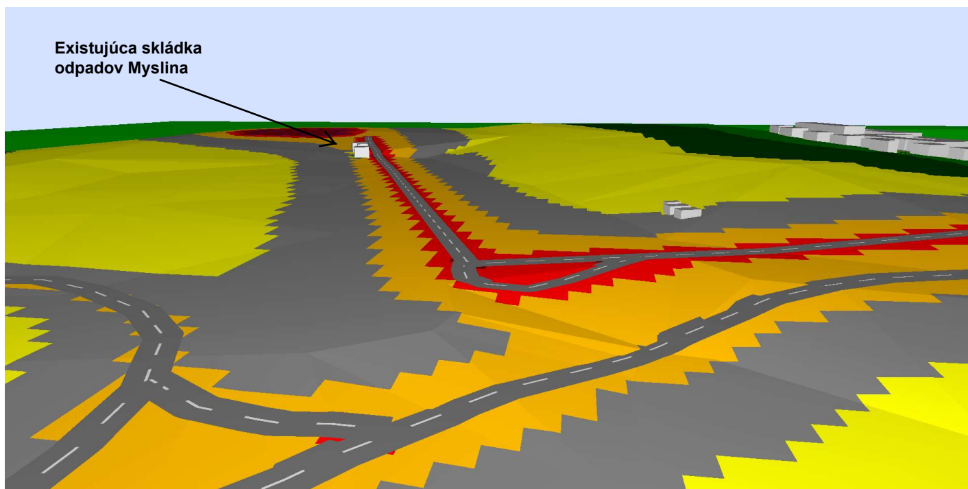
Príloha 1A - 3D pohľad matematického modelu (hlukovej mapy) záujmového územia "Skládka odpadov Myslina – Lúčky – CENTRUM MBÚ – Myslina" - denný čas - súčasný stav.
